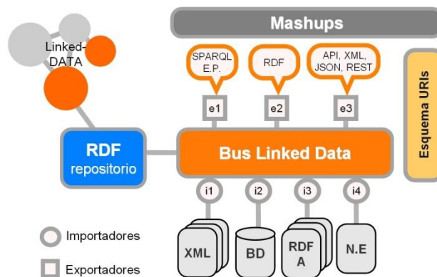
GRÁFICO IV.4 ARQUITECTURA GENERAL DE UN SISTEMA DE LINKED GOVERNMENT DATA
